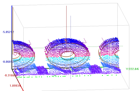
Abb. 2: 3D-Screenshot eines Coils in der Seitenansicht
